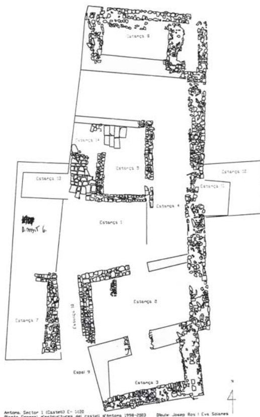
Antona. Sector I (Castell) E-1030 Planta General d'estructures del castell d'Antona 1998-2003. Dibuix Josep Ros i Eva Solanes
